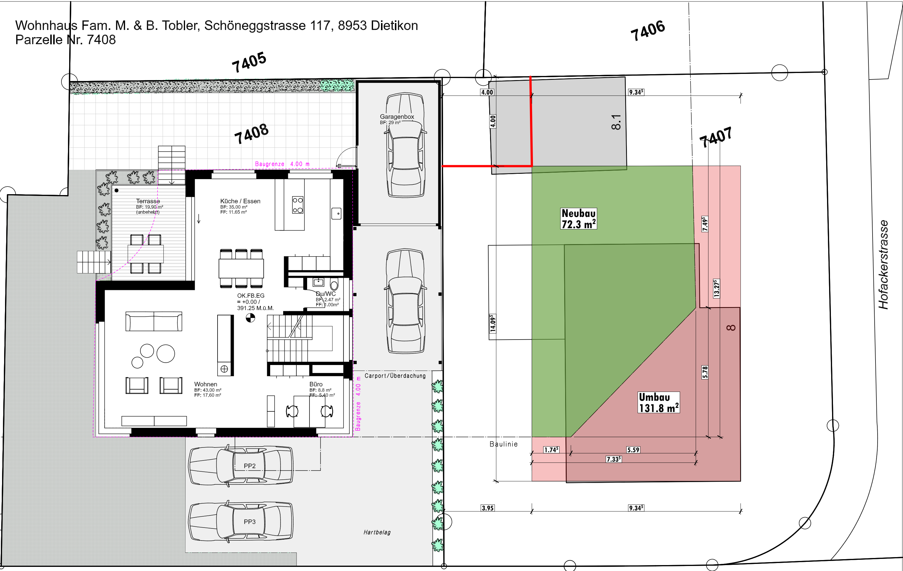
SITUATION / GRUNDRISS ERDGESCHOSS
